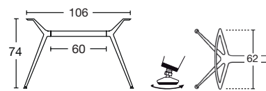
basamento con traversa corta base with short cross bar
