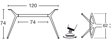
basamento con traversa lunga base with long cross bar
