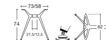
basamento con traversa mini base with mini cross bar
