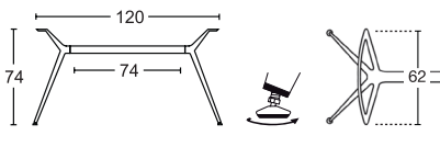
basamento con traversa lunga per piano cm 180x90 base with long cross bar for 180x90 top
